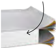
Isolierte Seitenwände/ Türelement Sandwichelement mit 40 mm Kern aus Styropor (EPS W20)
